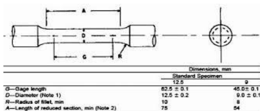
Gambar 32. Spesimen uji tarik standart ASTM E8
