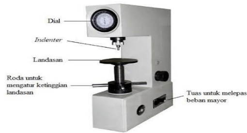
Gambar 29. Alat uji kekerasan
