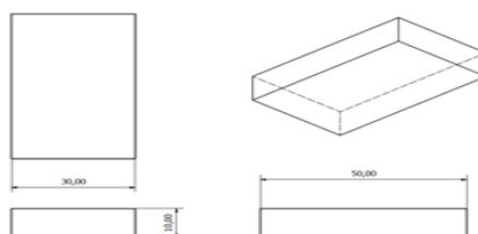
Gambar 33. Spesimen uji kekerasan
