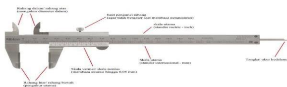
Gambar 17. Jangka Sorong
