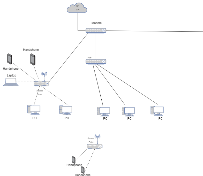
Gambar 22. Topologi jaringan Balai Kampung Rama Klandungan. (Sumber: Penulis, 2023)
